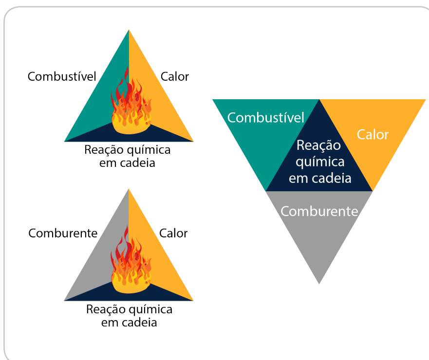
Figura 2 - Tetraedro do Fogo
