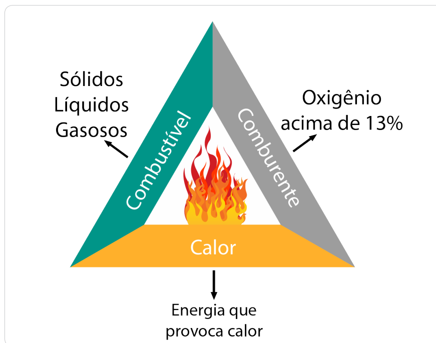
Figura 1 - Triângulo do Fogo
