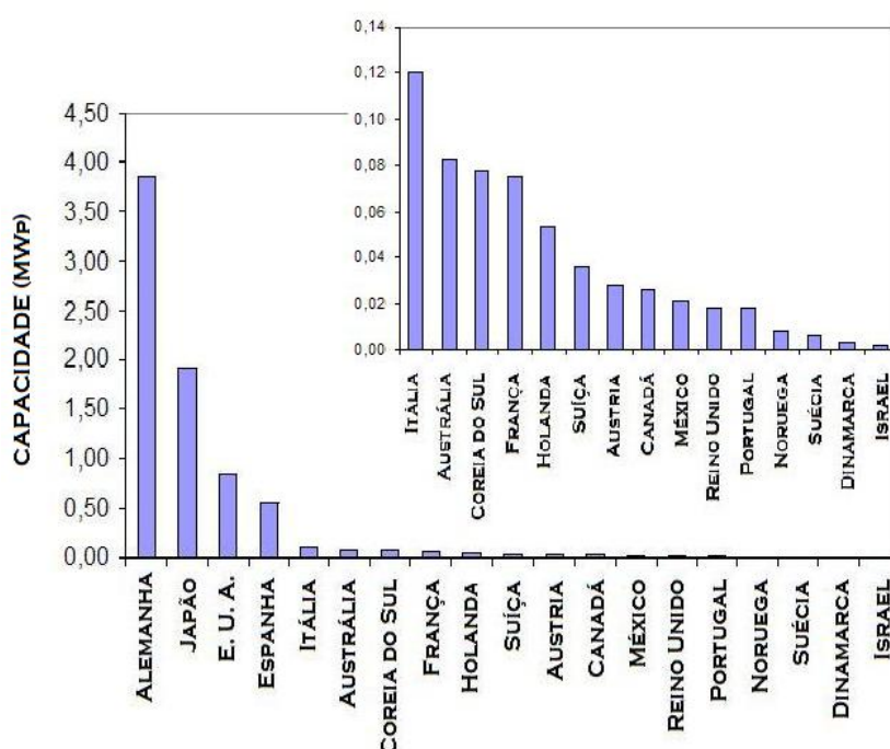
Figura 2a. Capacidade total instalada (MW) nos 15 maiores produtores mundiais de energia fotovoltaica. Fonte: Adaptado do relatório da International Energy Agency 10
